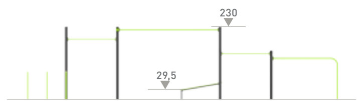
ELEWACJA
